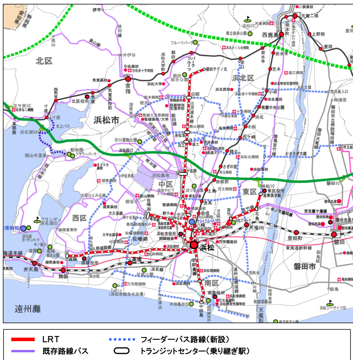
図 4-18 LRT路線構想(案)とフィーダーバス乗り継ぎ関係図
