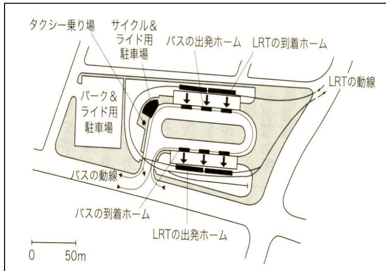
図 6-9 ミニバスターミナル(ドイツ・ハノーファ市の例)
