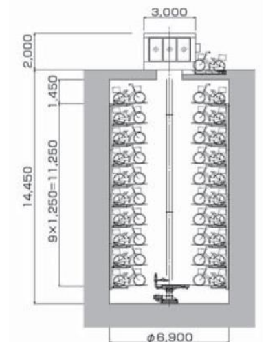
図 7-18 立体式の構造
